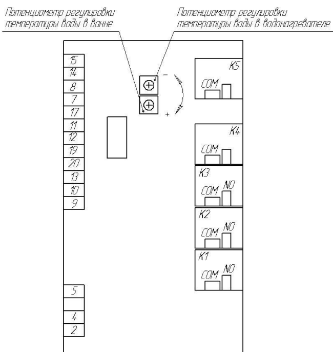
Рисунок 2 – Условное обозначение контактов блока управления
