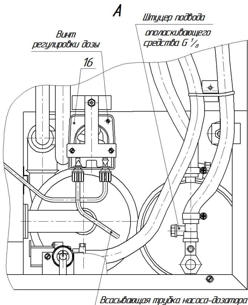
Рисунок 1 (лист 2 из 2) – Машина посудомоечная фронтальная МПФ-30-01
